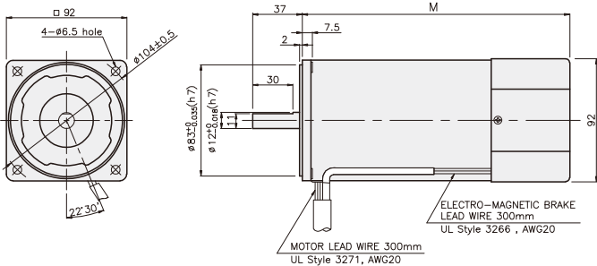
尺寸表
